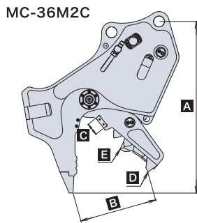
■MC小割機 with マグ・ゴン 仕様図
