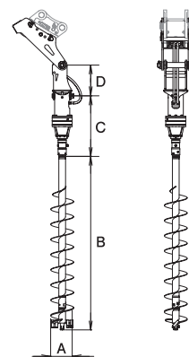
■ミニアースオーガー 仕様表
