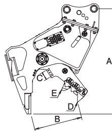
■ MC小割機 with マグ・ゴン SPシリーズ 仕様表
