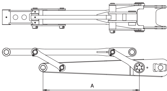
■マルチエクステンションアーム 仕様図
