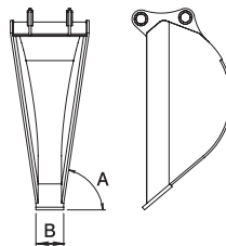
■暗渠バケツ TB 仕様表
