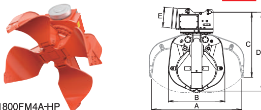
■オレンジバケット with マグ・ゴン仕様表
