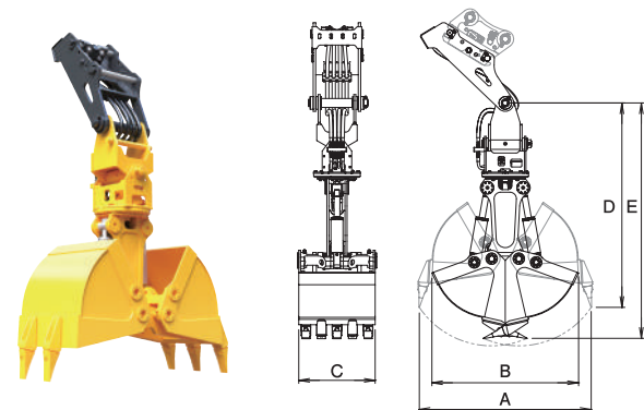
■全回転クラムシェルバケット 仕様表
