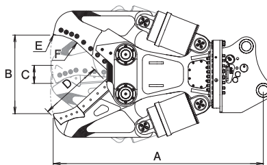
■DXカッター 仕様図
