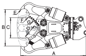
■DX-SRC/DI-SRC大割Cutter S/A/ASタイプ 仕様表
