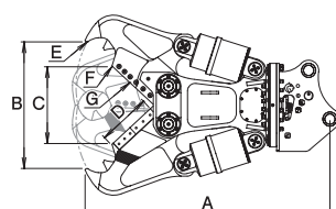
■DX-SRC/DI-SRC大割Cutter S/A/ASタイプ 仕様表
