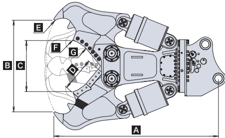
■DX-SRC大割カッター 仕様図
