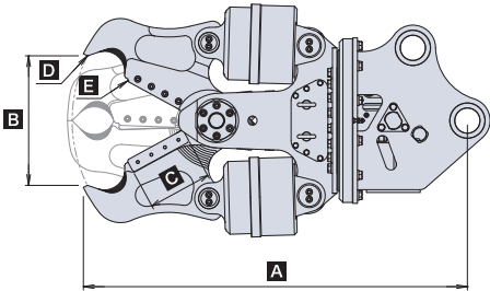
■DF大割カッター 仕様図
