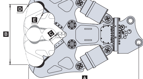
■D大割機 仕様図
