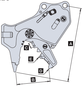
■MC小割機 with マグ・ゴン 仕様図
