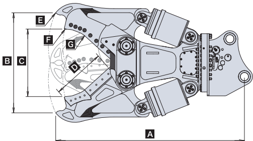
DXGGカッター 仕様図
