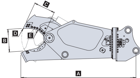
■GSシャー 仕様図
