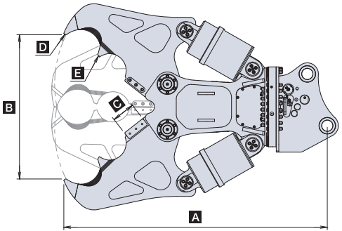
D大割機 仕様図
