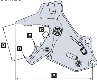
■MC小割機 with マグ・ゴン 仕様図
