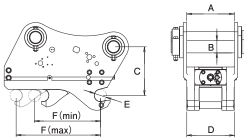
■機械式ワンキャッチ 仕様図
