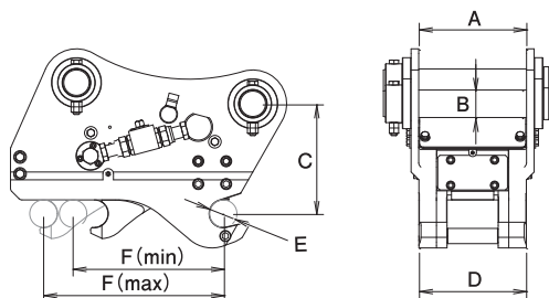
■油圧式ワンキヤッチ 仕様図
