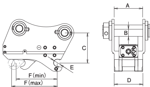
■機械式ワンキヤッチ 仕様図
