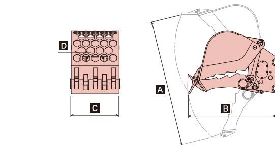
■CBRH-L(ハニカムスケルトン仕様) 仕様図
