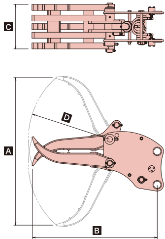
■首振りグラスパーVL 仕様図
