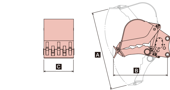
■CBRB-L(バケット仕様) 仕様図
