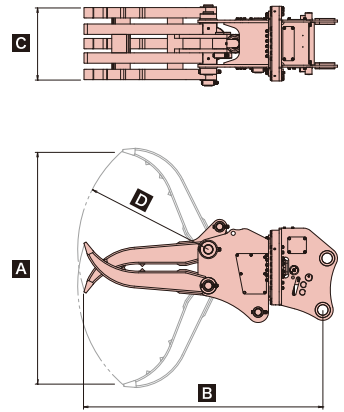
■ハイブリッド 全旋回グラスパー SSD 仕様図
