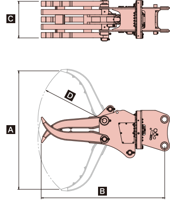
■全旋回グラスパー ソル 仕様図
