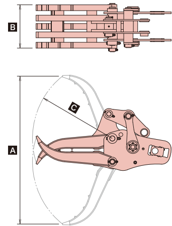
■グラスパーV3 仕様図
