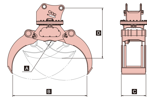
■全旋回木材グラスパー 仕様図
