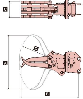
■全旋回グラスパー ダイナ 仕様図
