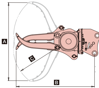
■ マグ・ゴン 全旋回グラスパー 仕様図
