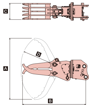
■ハイブリッド 全旋回グラスパー SSC 仕様図
