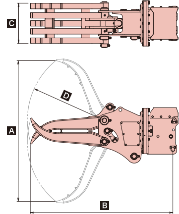
■完全油圧式ワンキャッチ専用 全旋回グラスパー 仕様図
