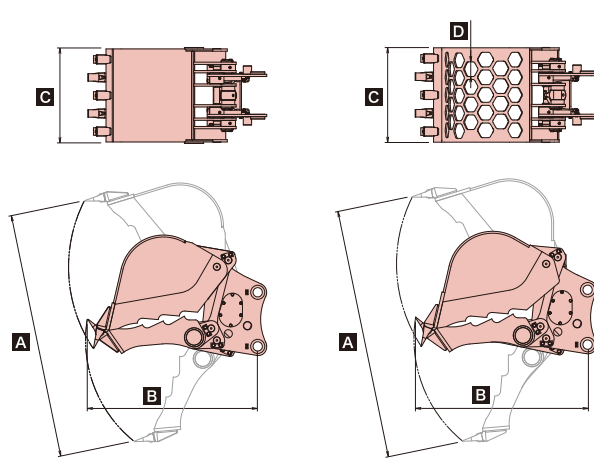
■ CBRB(バケット仕様)仕様図
