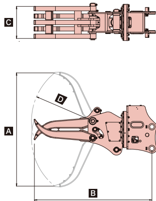
■全旋回グラスパー ダイナ 仕様図
