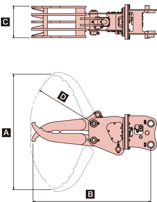
■全旋回グラスパー ソル 仕様図
