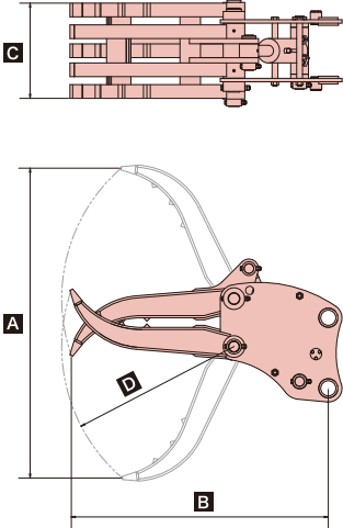
■首振りグラスパーVL 仕様図
