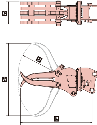
■全旋回グラスパーVS 仕様図
