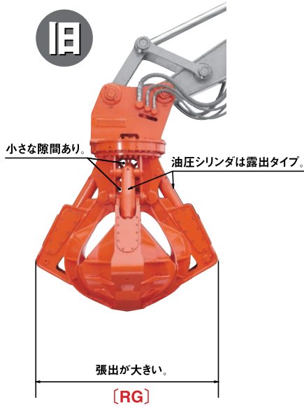
旧型オレンジバケットRG (RP)
